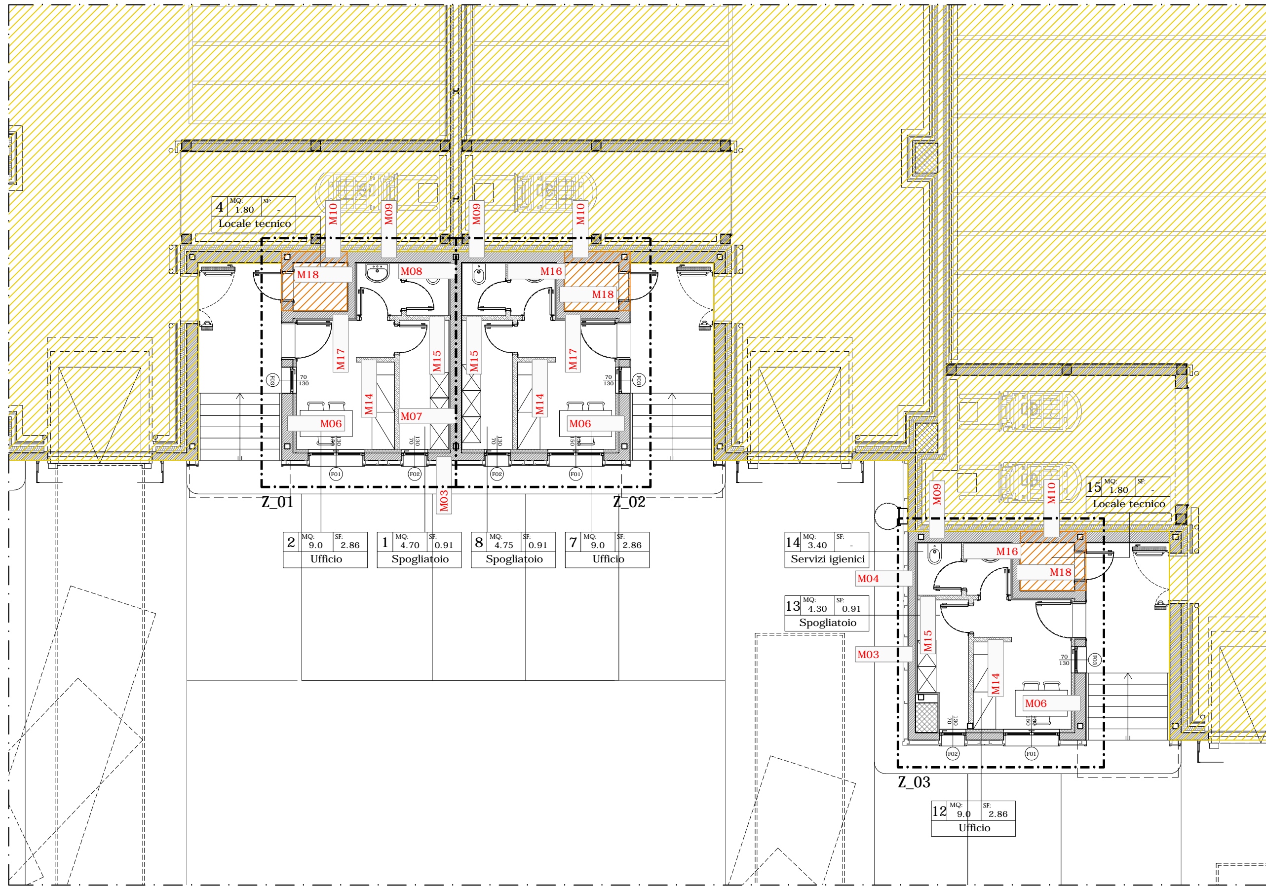
Stralcio Planimetria Uffici Blocchi 1, 2, 3 - Rapp. 1:100
