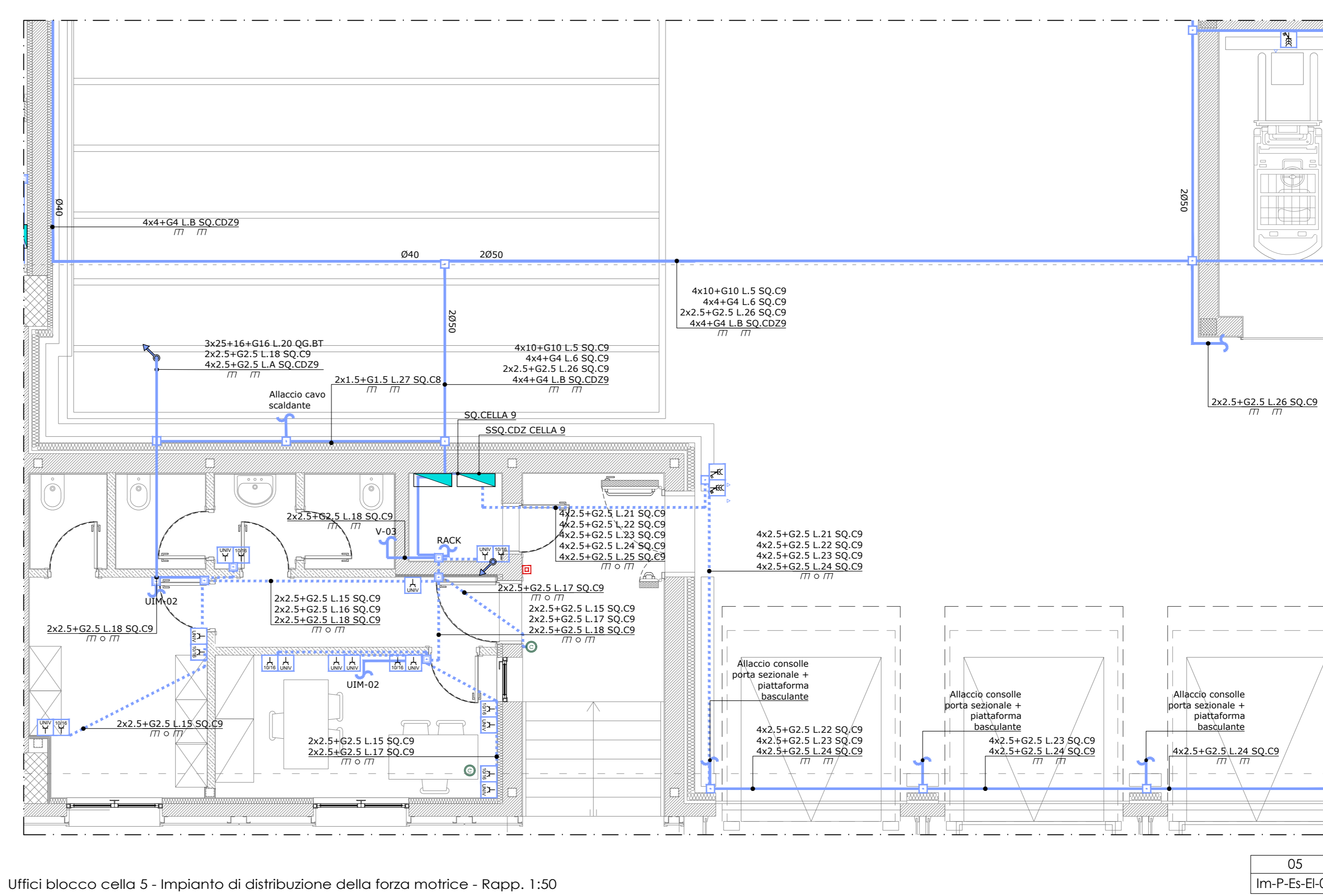
Uffici blocco cella 5 - Impianto di distribuzione della forza motrice - Rapp. 1:50
