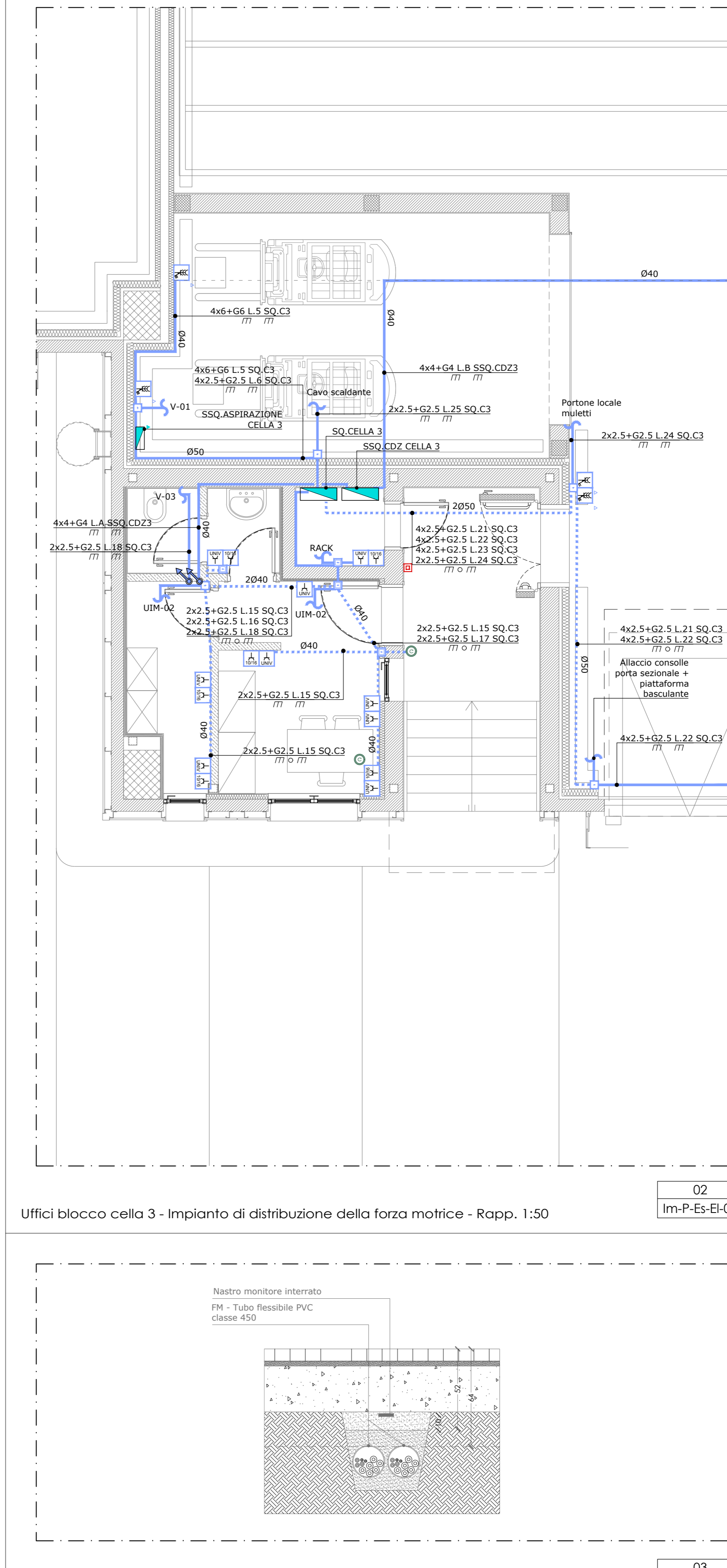
Posa cavidotti interni - Rapp. 1:20
